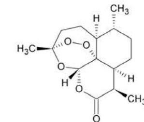
Artemisinin
