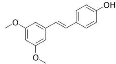
Pterostilbene
