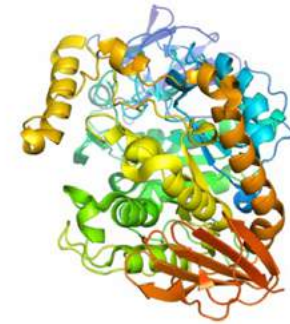
Amylase
