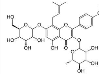
Icariin
